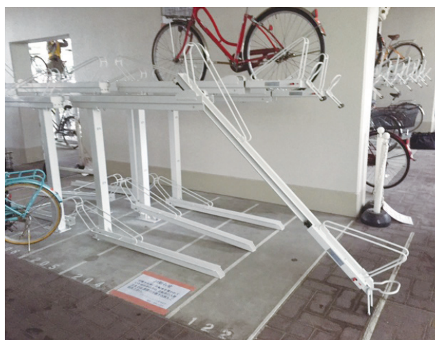
OE-G型 着地式タイプ
