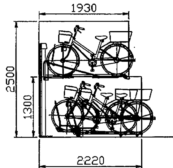
垂直2段式駐輪機 CS2AF-2A10型
