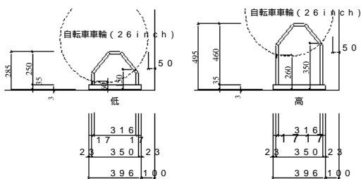
標準側面図 S = 1 / 4 0
