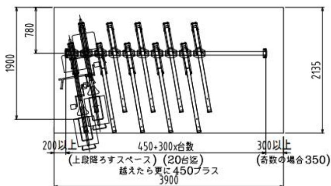
下段前後入れ(AB10)平面図
