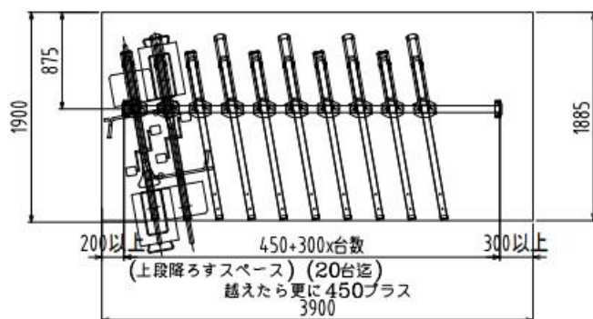
下段前後入れ(AB10)平面図
