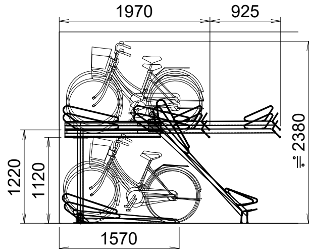
固定2段式 OE-TG型 (単独柱 着地式)
