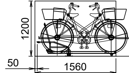
スライド式平置きC-AB30型 (前入れのみ電動アシスト車対応)
