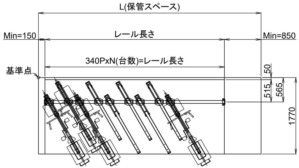
平面図
