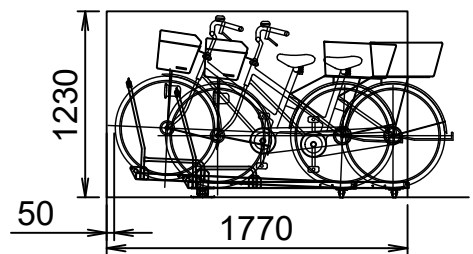
スライド式平置きC-2A30型 (電動アシスト車対応)
