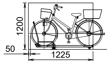
スライド式平置きC-1A45型 (電動アシスト車対応)
