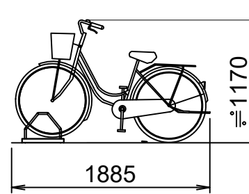
固定式前輪ラックOE-ZM型 (単独ベース)
