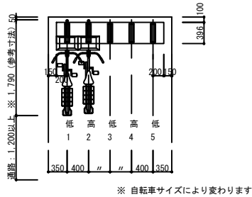
標準平面図 S=1/100
