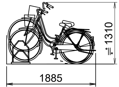
固定式前輪ラックOE-ZM型
