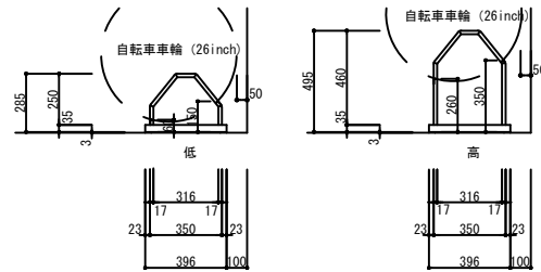
標準側面図 S=1/40
