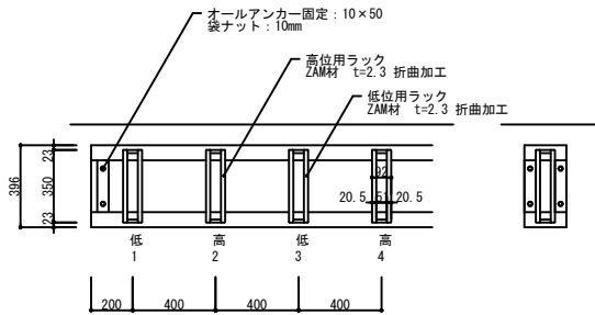
標準平面図 S=1/40
