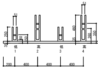
標準正面図 S=1/40
