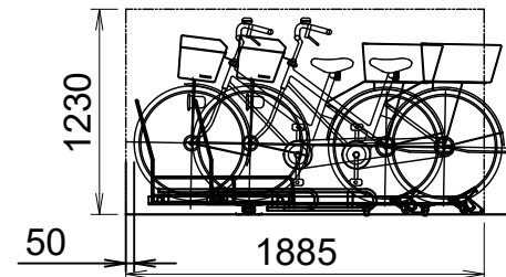
スライド式平置きC-2A30C型 (カート式) (電動アシスト車対応)
