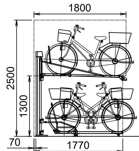
垂直2段式 CS2R-AB30型
