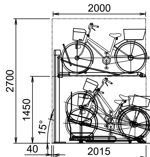
垂直2段式 CS2AFH-HL10C型 (カート式)
